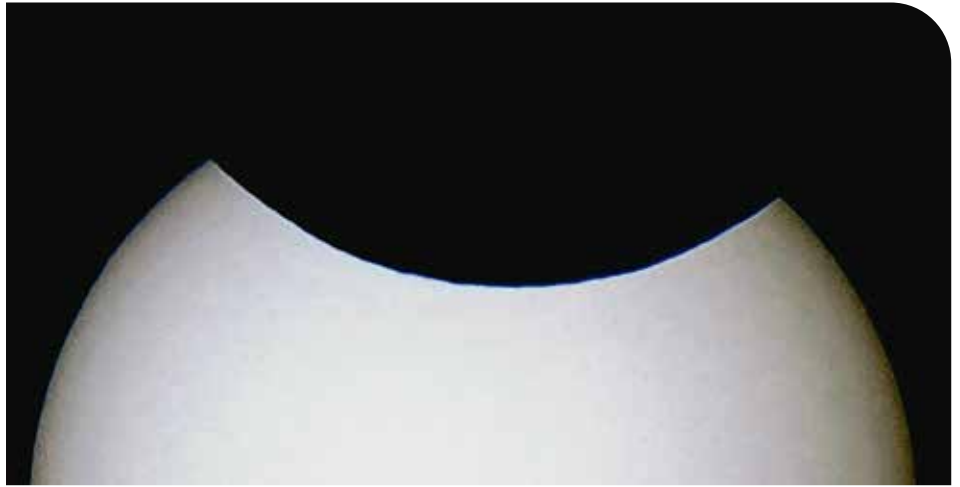
Die Sonnenfinsternis am 10. Juni 2021
