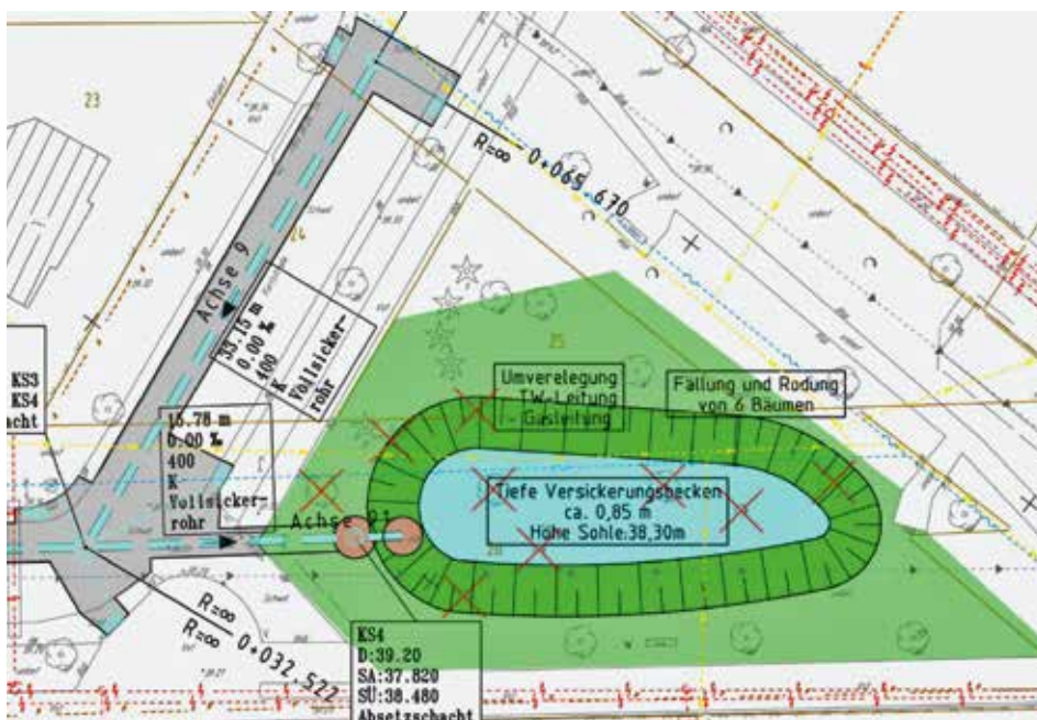
Vorentwurf Neubau Entwässerung Dr. Löber
