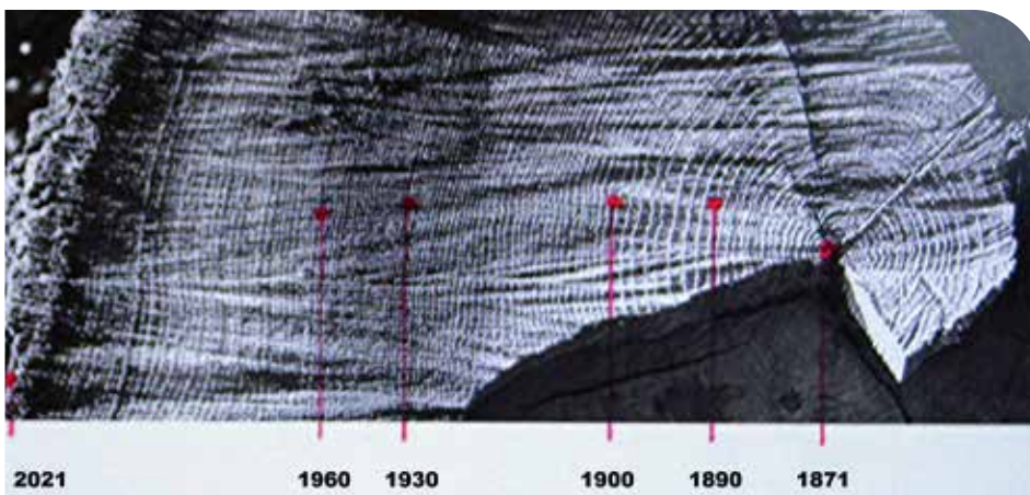
Baumringe, entstanden in 150 Jahren.
