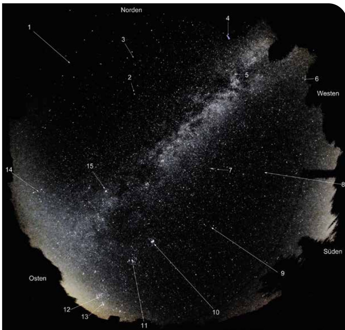
Die Milchstraße und ihre Sternbilder Foto: Jörg Meyer
