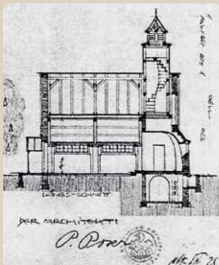
Bauzeichnung der Kapelle von P. Poser (September 1925) Quelle: Archiv Autor
