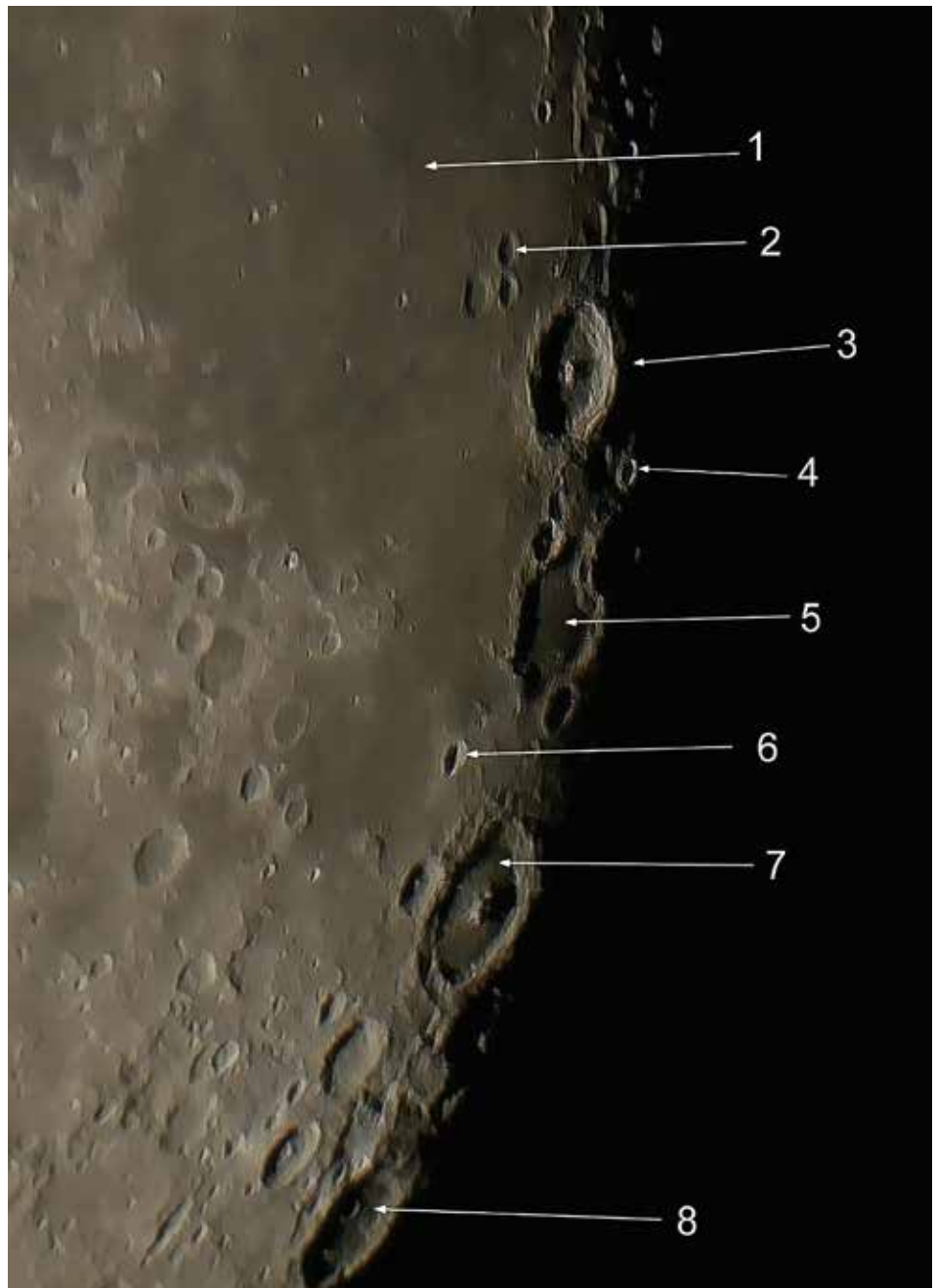
Aufnahme vom 25. August 2021 um 03:44 Uhr mit 200-mm-Öffnung und 4-Meter-Brennweite – das kleinste Detail ist etwa 3 bis 5 Kilometer groß.
