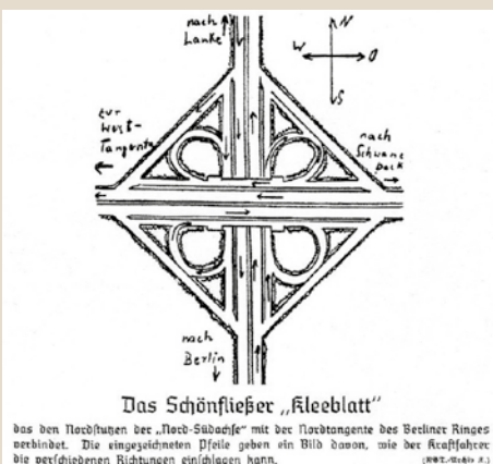
Bild 2: Handskizze zum Schönfließer
